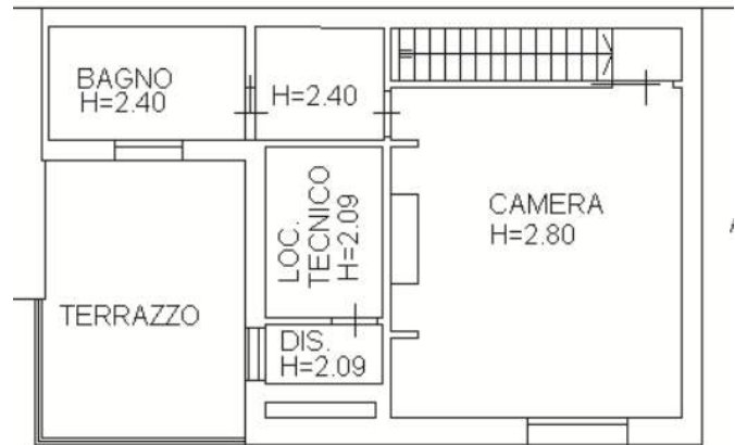
PIANO PRIMO
